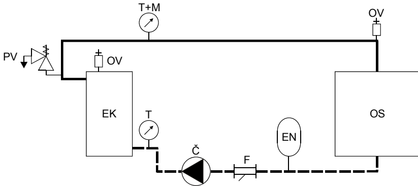
Vytápěcí systém s nuceným oběhem
