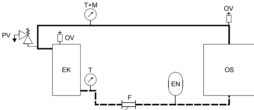
Vytápěcí systém se samotížným oběhem
