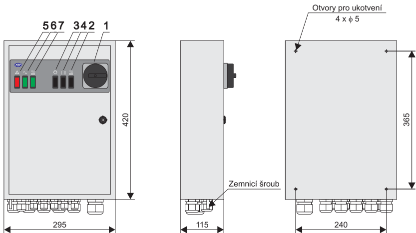
Ovládací skříňka elektrokotle
