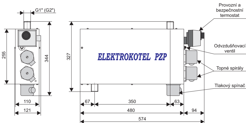
Elektrokotel PZP - MINI
