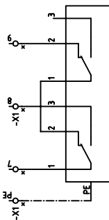
Bezpečnostní termostát elektrokočle
